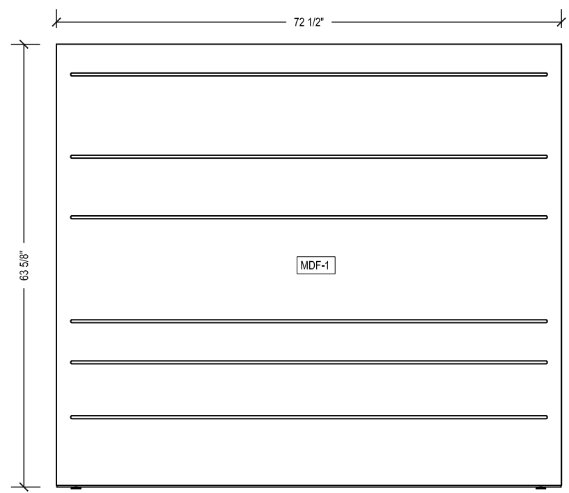
5 ELEVATION SCALE: 5/8" - 1'-0"
